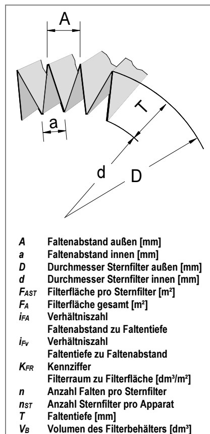
Abb. 1: Abmessungen am Sternfilter
