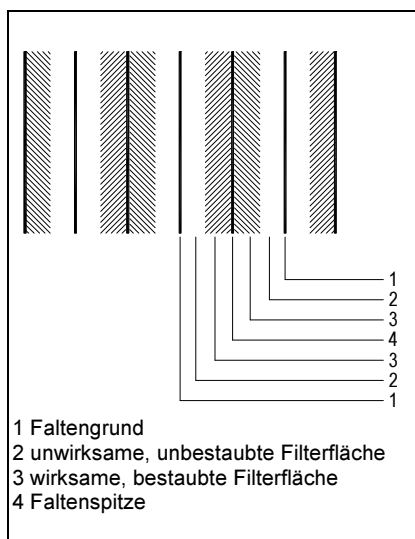
Abb. 2: Abwicklung eines gebrauchten Sternfilters
